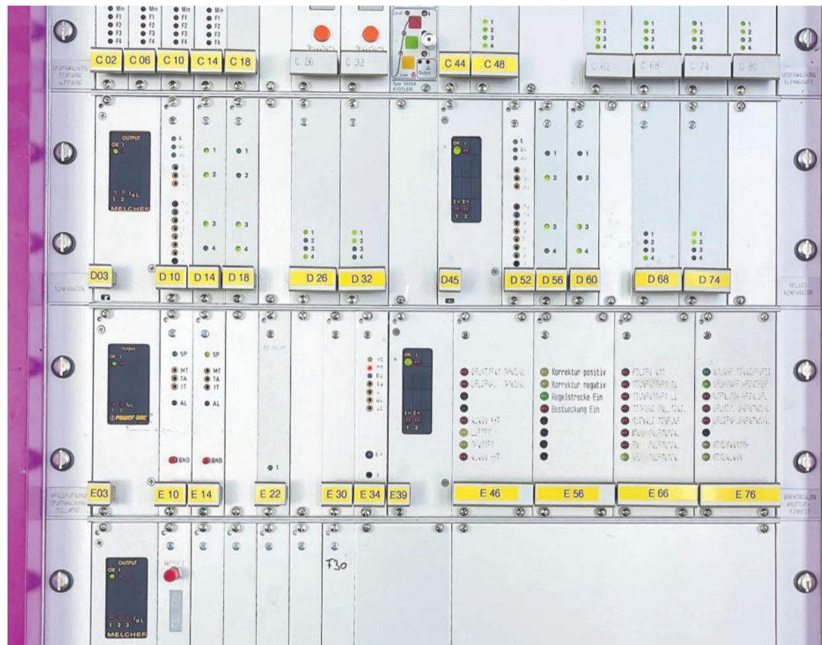
Der Schaltschrank des Sesselliftes Mot da Ri. Die schwarzen Felder sind Melcher-Transformatoren. Foto: Melcher
